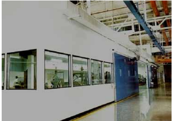
隔声室在工厂的应用 哪怕厂房内的噪声90分贝，隔声室内可保持50分贝以下的环境
